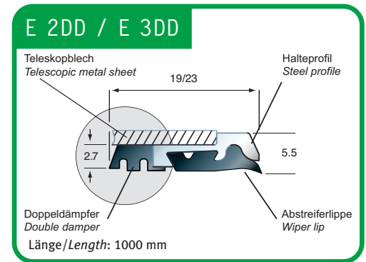
Abstreifer eingebaut gezeichnet. Wipers shown in mounted position.
